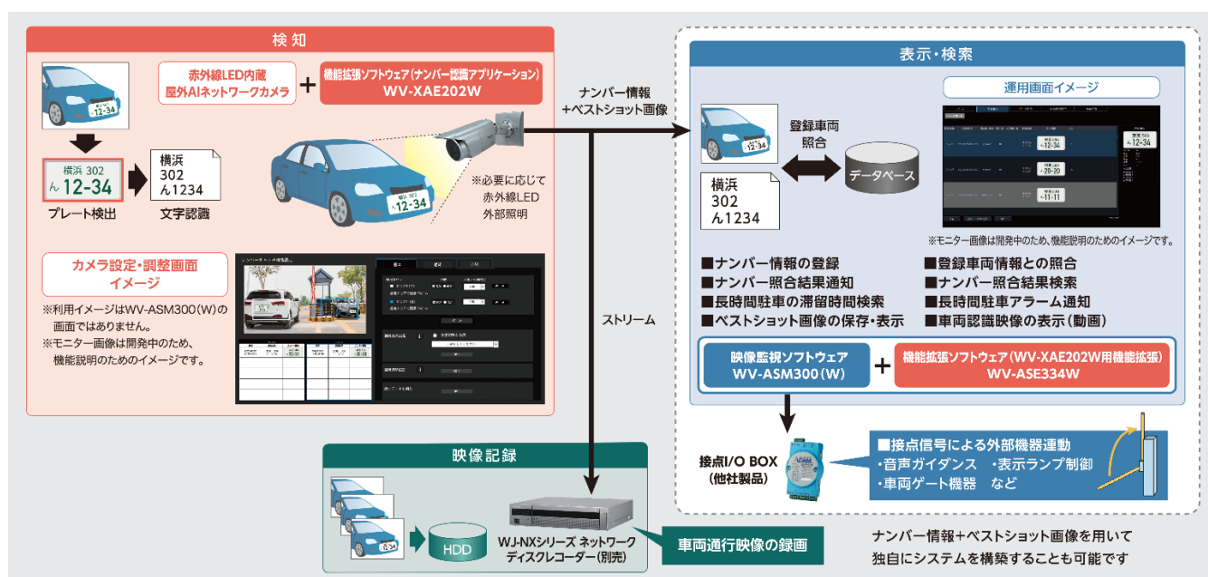
NumberCATCH II のシステム構成イメージ
