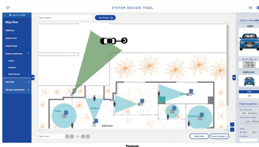
システムデザインツールのシミュレーション・ガイドの画面
